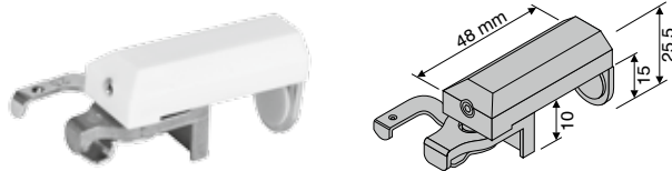
Klemmträger mit Schnellspannung
