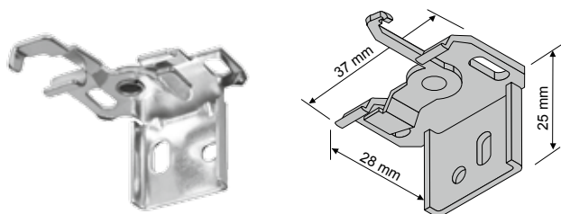
Wand- / Deckenträger mit Schnellspannung
